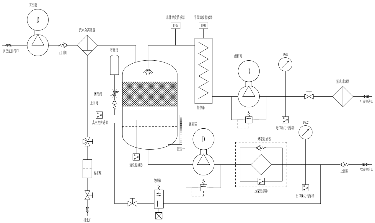
系统管线图
